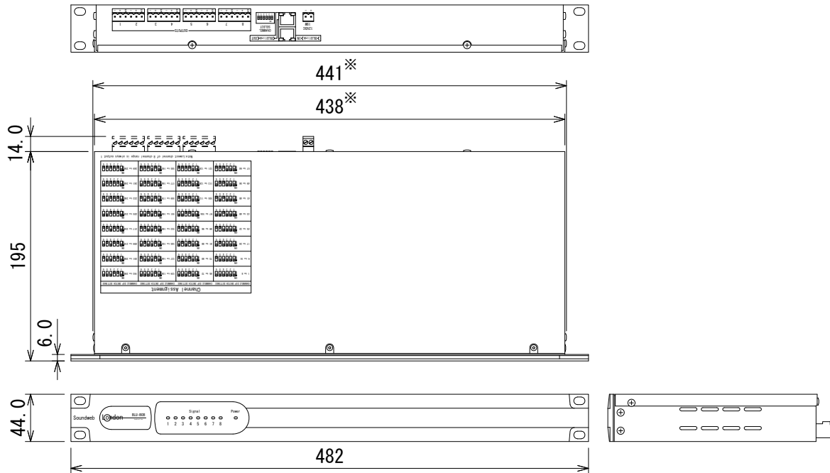
背面図のみユーロブロック非装着状態
