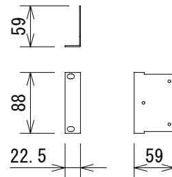
ラックマウント金具 (付属品)
