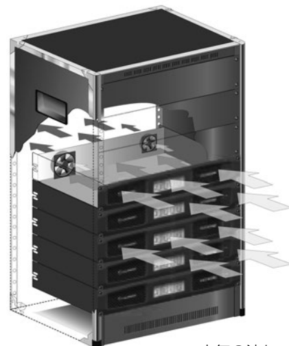
空気の流れ
