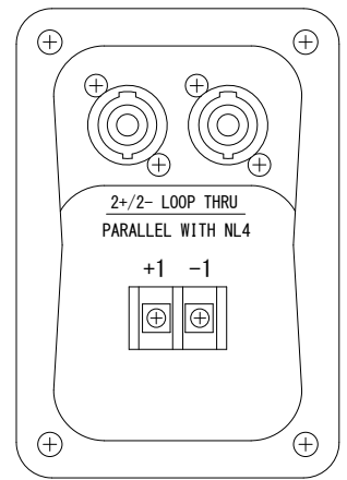
背面端子拡大図
