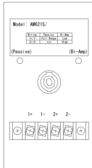
端子拡大図
