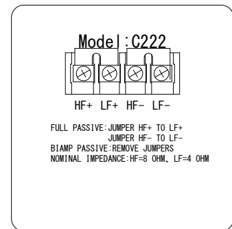
側面端子拡大図
