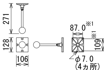
壁取付金具
