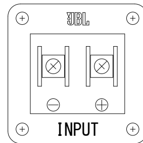
端子拡大図
