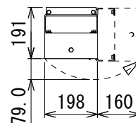
メンテナンス時の金具回転必要寸法 (左右に回転可)
