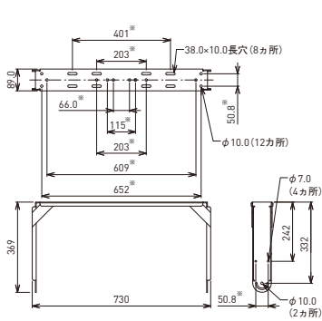
AW266、AW295
