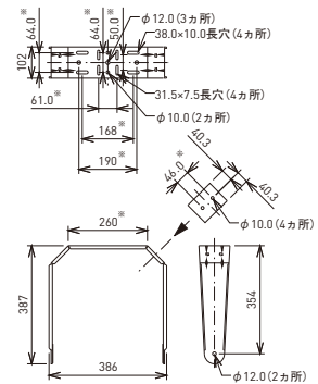
AWC129
