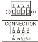
端子拡大図
