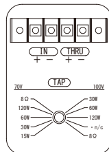
端子拡大図
