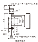
壁取付金具
