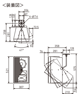
※スピーカーを縦に取り付ける場合は、高域ドライバーを下向きで使用してください。
