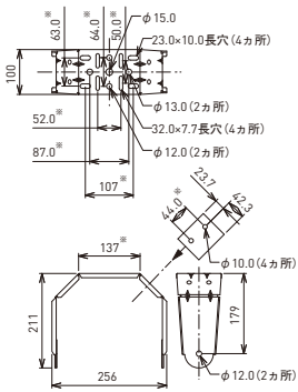
AW266、AW295
