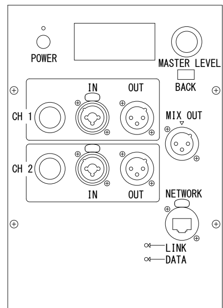
コネクターパネル拡大図
