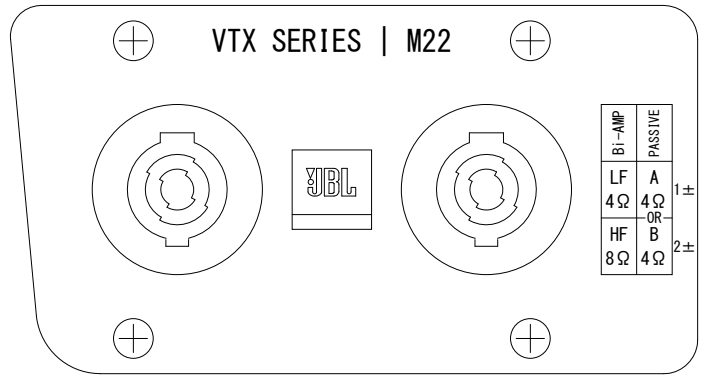
コネクターパネル拡大図
